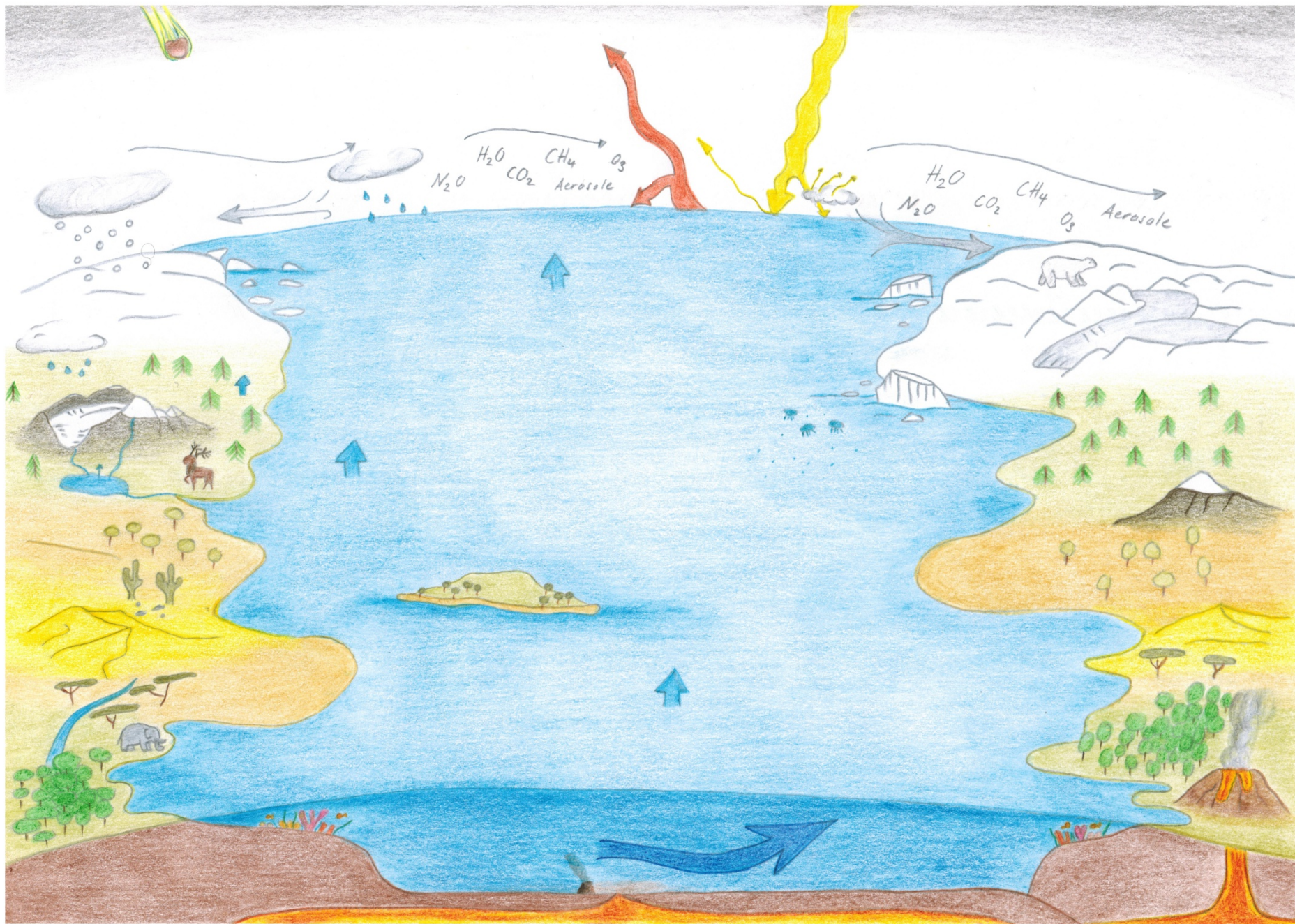
Fig. 2 Système climatique naturel
