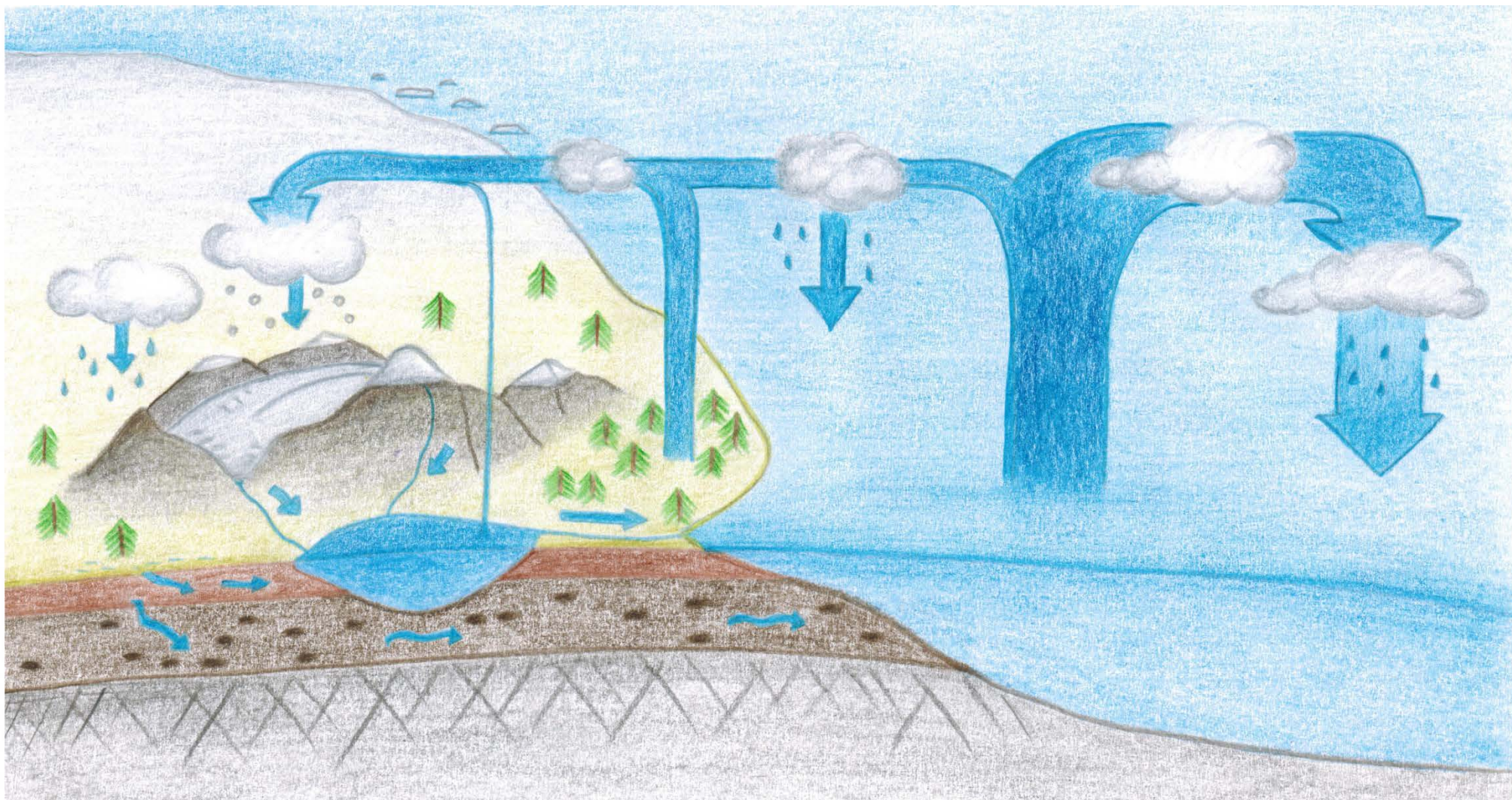
Fig. 6 Cycle de l'eau
