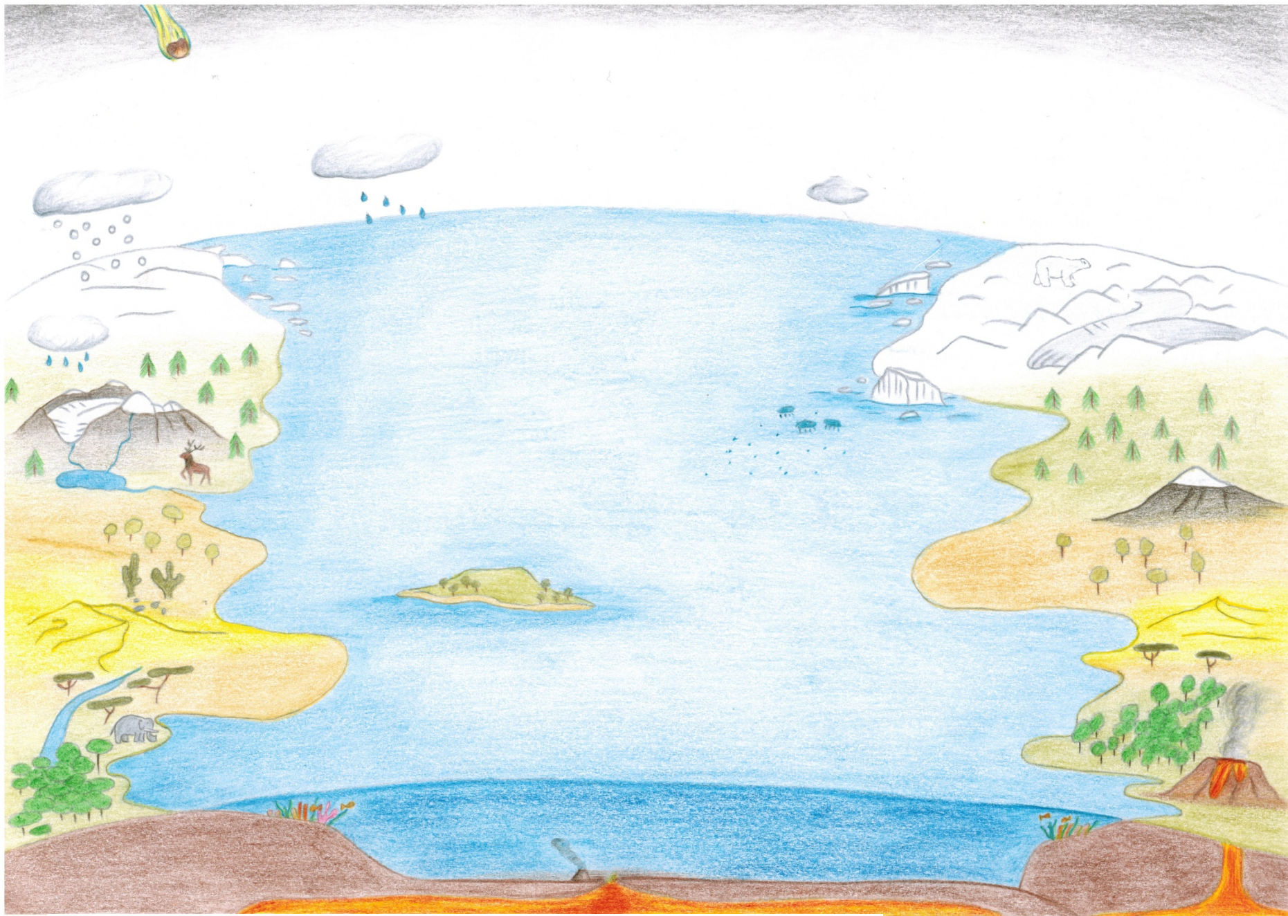
Fig. 1 Système climatique naturel (sans les différents types de rayonnement et de flux)
